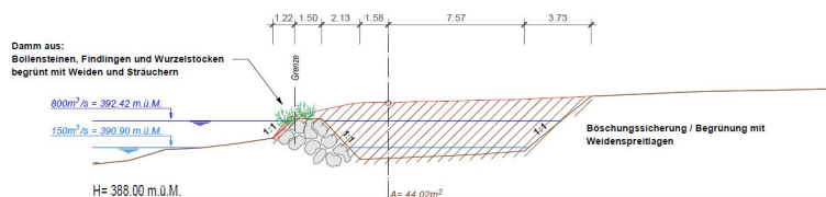
Querschnitt Nr.5 Grundstück Gemeinde 1:200
