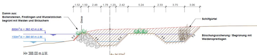
Querschnitt Nr.6 Grundstück Gemeinde 1:200
